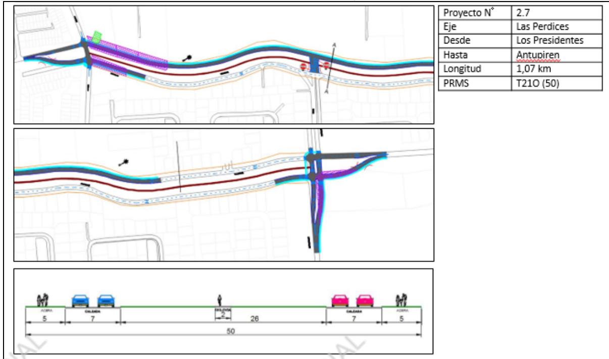
FIGURA N° 2-32. Prediseño 2.7: Las Perdices, Habilitación Doble Calzada.
