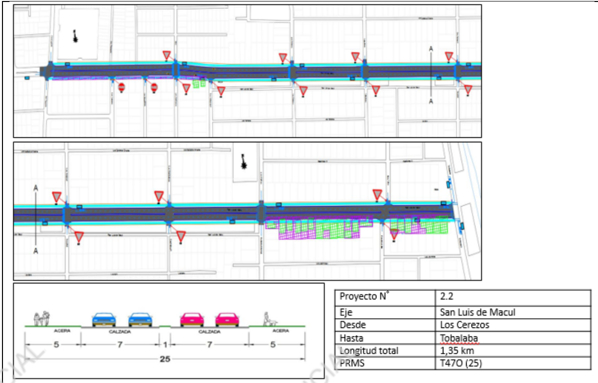
FIGURA N° 2-27. Prediseño 2.2: San Luis De Macul, Habilitación Doble Calzada.
