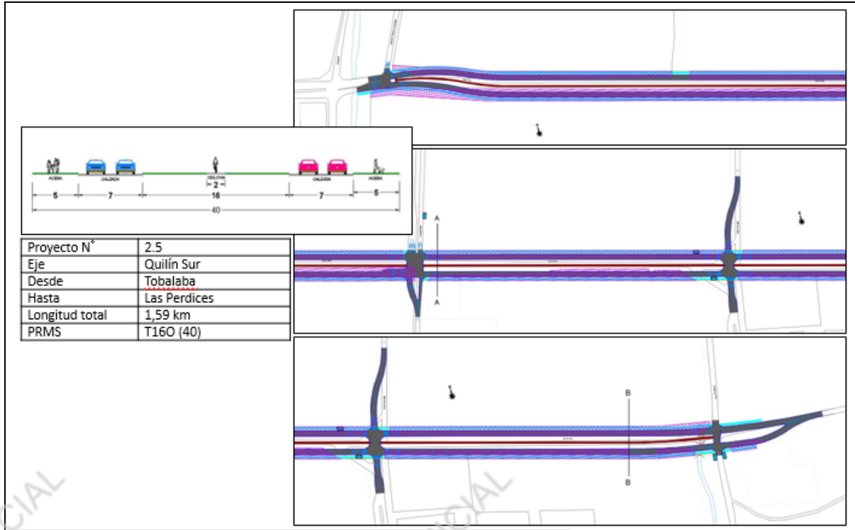
FIGURA N° 2-30. Prediseño 2.5: Quilín Sur, Habilitación Doble Calzada.
