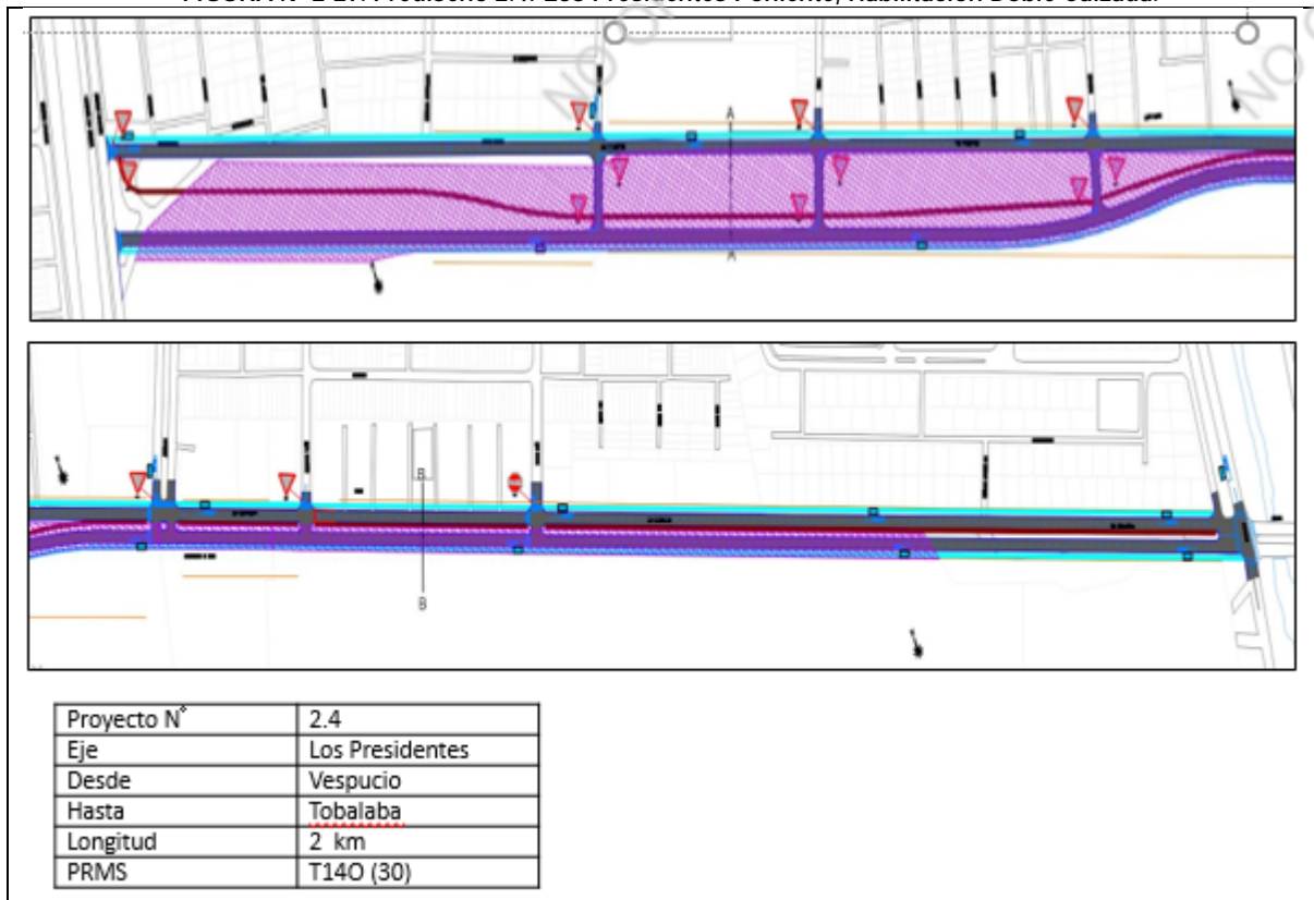
FIGURA N° 2-29. Prediseño 2.4: Los Presidentes Poniente, Habilitación Doble Calzada.
