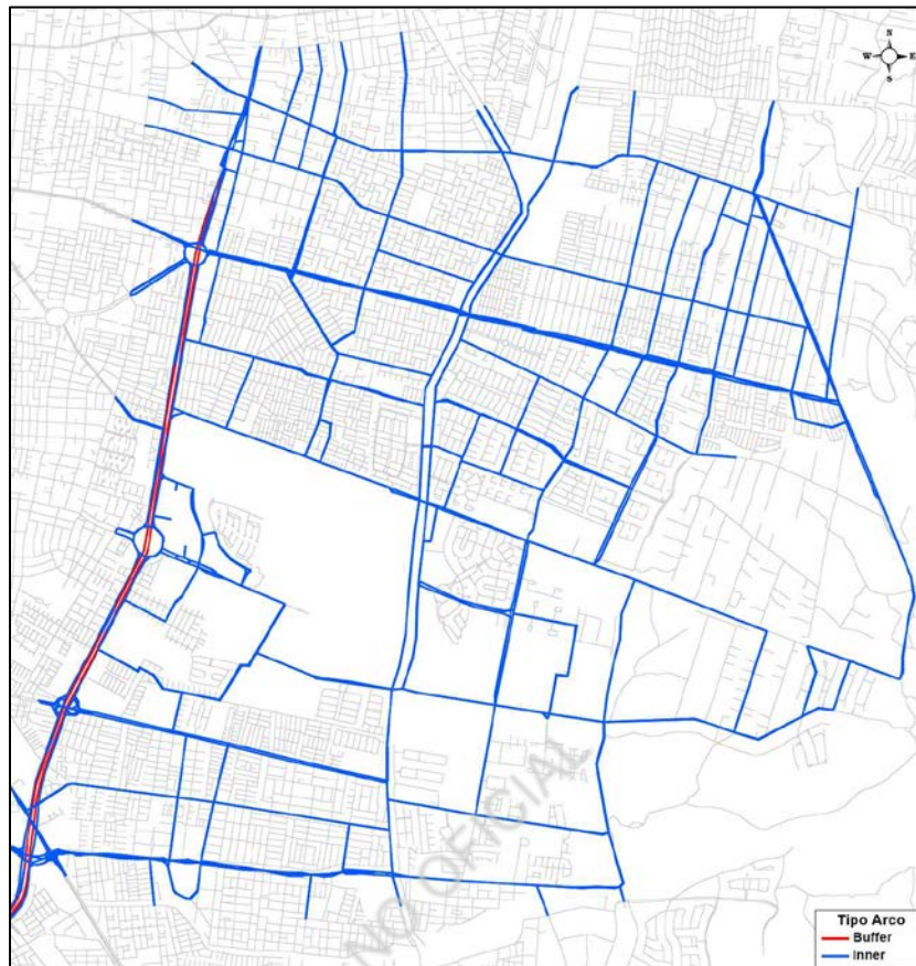
FIGURA N° 2-12. Red de modelación SATURN, Calibración año 2014, Periodo Punta Mañana, Sector comuna de Peñalolén
