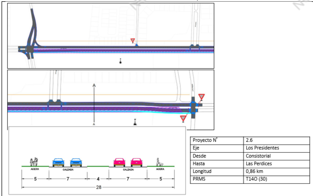
FIGURA N° 2-31. Prediseño 2.6: Los Presidentes Oriente, Habilitación Doble Calzada.
