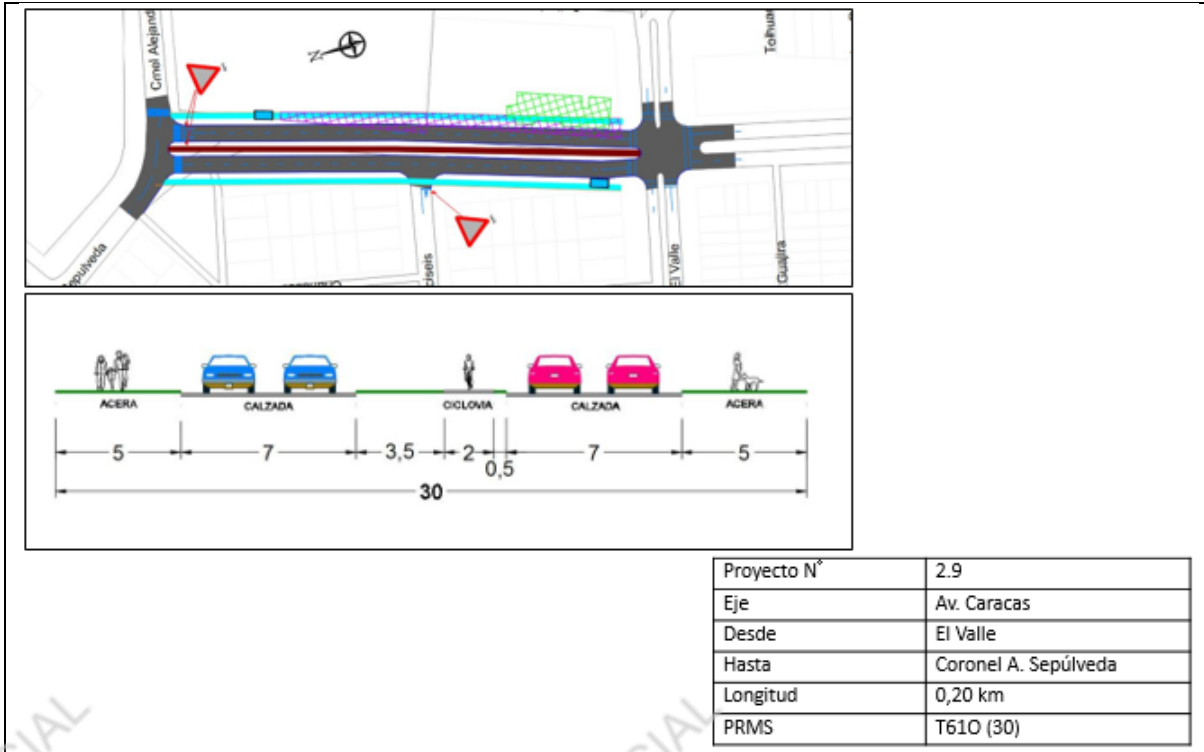
FIGURA N° 2-34. Prediseño 2.9: Avenida Caracas, Habilitación Doble Calzada.
