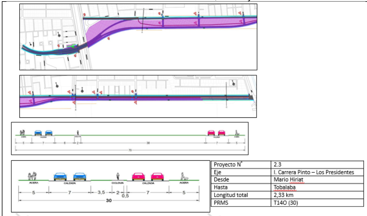
FIGURA N° 2-28. Prediseño 2.3: Conexión I. Carrera Pinto, Desnivel y Habilitación Doble Calzada.
