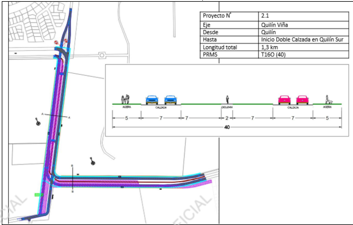
FIGURA N° 2-26. Prediseño 2.1: Quilín Viña, Habilitación Doble Calzada.
