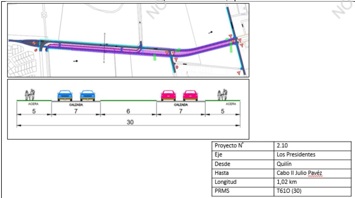
FIGURA N° 2-35. Prediseño 2.10: Apertura Los Cerezos, Apertura Doble Calzada.
