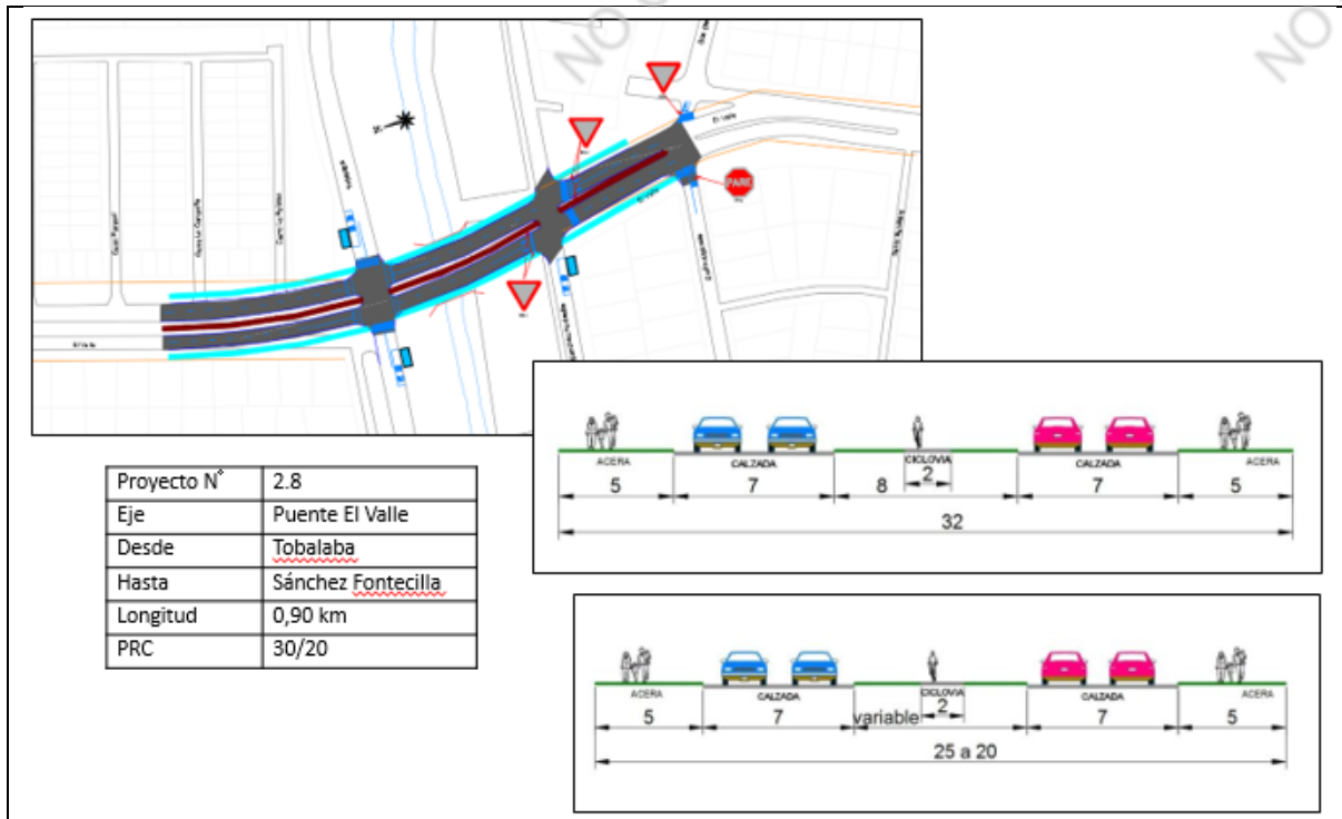
FIGURA N° 2-33. Prediseño 2.8: Puente El Valle.
