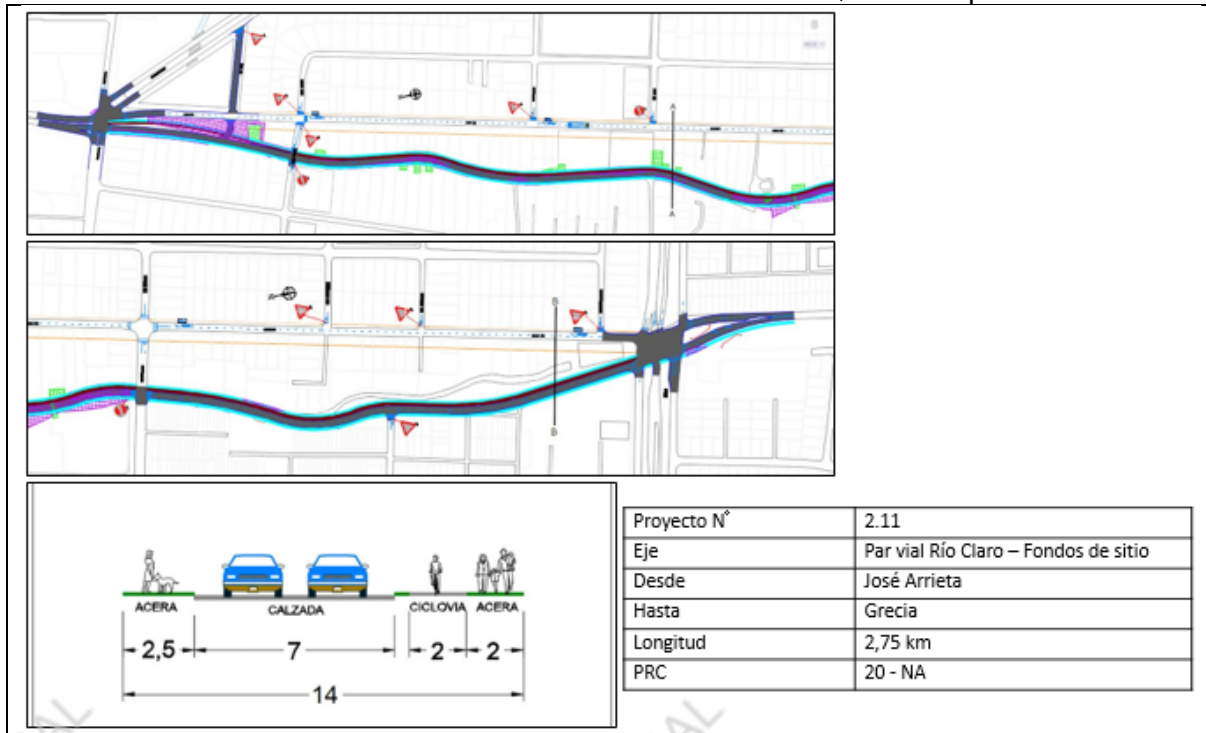
FIGURA N° 2-36. Prediseño 2.11: Par Vial Río Claro- Fondos de Sitio, Dos Pistas por Sentido.
